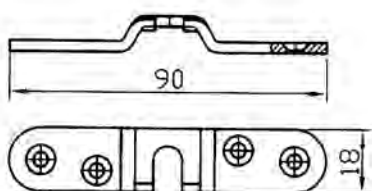
VKO ROBO NOSAČ KRILA 12.15-4
