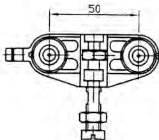
VKO ROBO DVOSTRUKA KOTURALJKA 12.15-2
