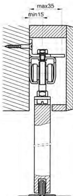
UČVRŠĆIVANJE NA BOČNU STRANU
