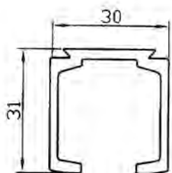
VKO ROBO TRAČNICA 12.15-1
