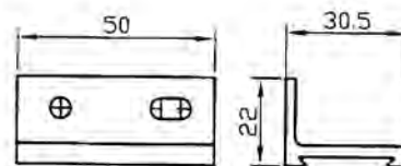
VKO ROBO NOSAČ TRAČNICE 12.15-3
