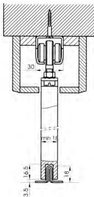
UČVRŠĆIVANJE NA HORIZONTALNU STRANU
