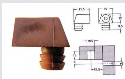
SPOJKA UTISNA S EKSCENTROM
