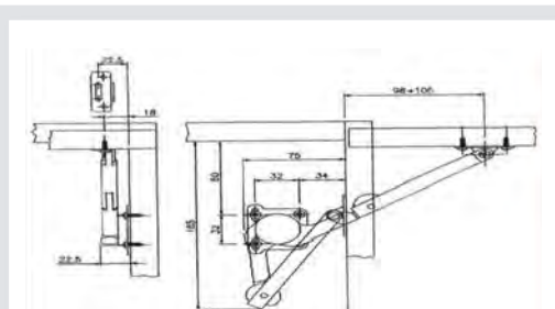
FGV - DRŽAČ DIZAJUĆIH VRATA S REGULATOROM BRZINE ZATVORENI
